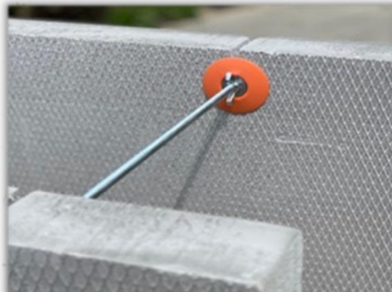
SPOJOVACÍ POZINKOVANÝ TŘMEN S KŘÍDLOVOU MATICÍ
